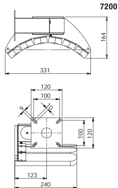
Flangia di fissaggio 120x120mm Fixing flange 120x120mm
